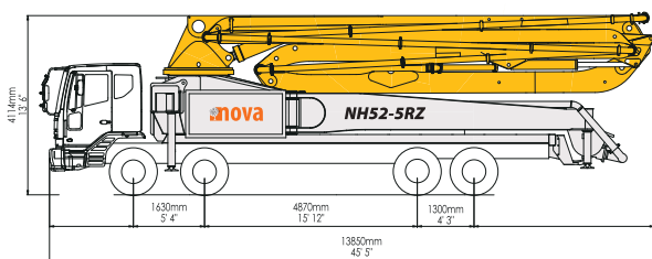
Dimensions
